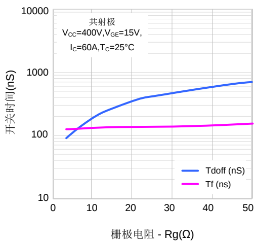
图10. 关断特性 vs. 栅极电阻
