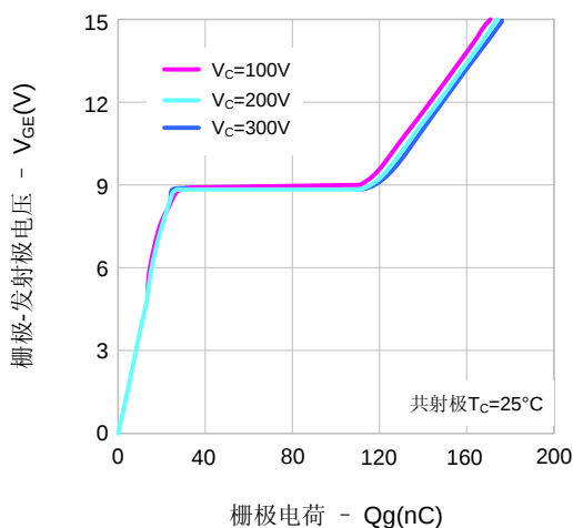
图8. 栅极电荷
